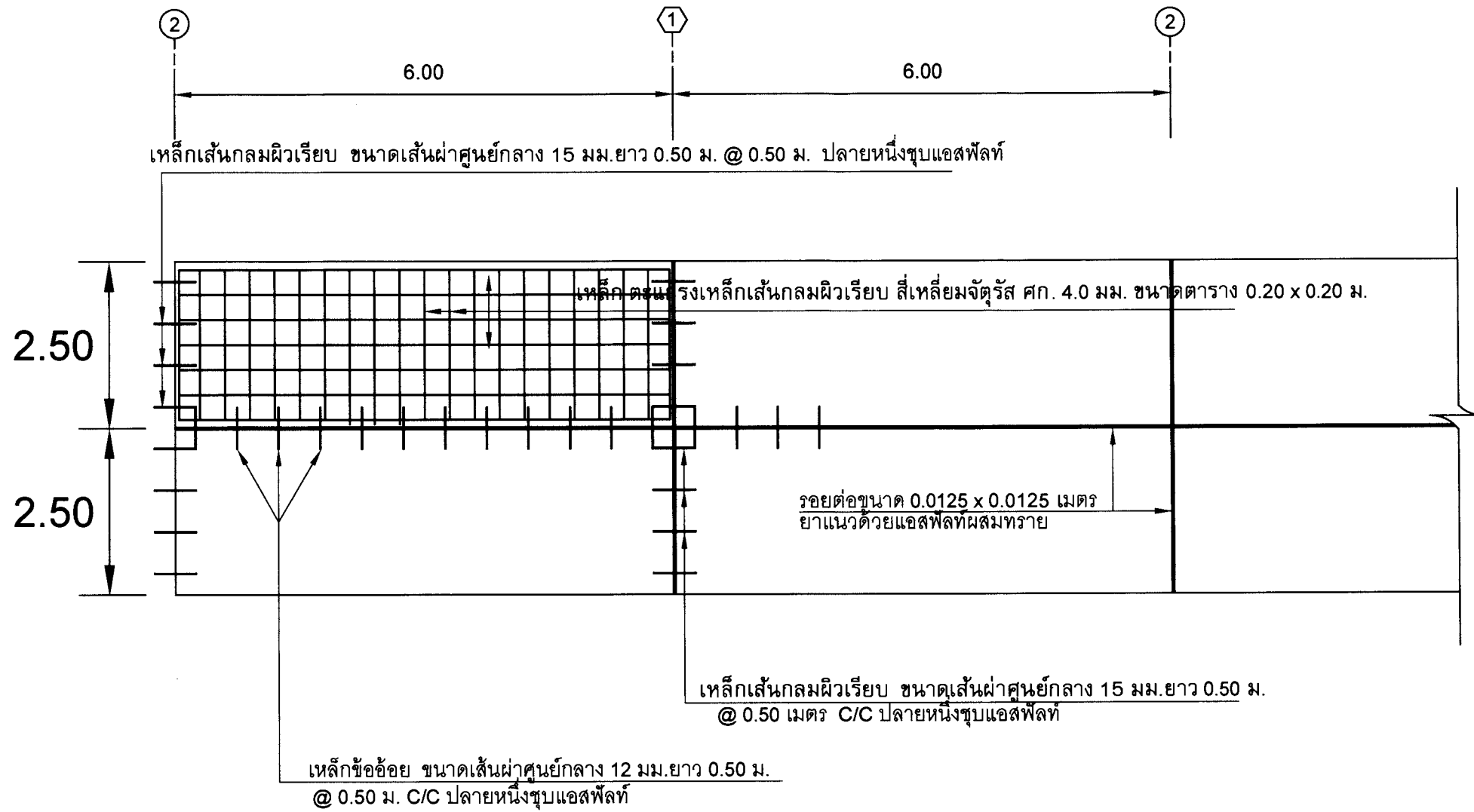
แปลนแสดงการผูกเหล็ก มาตราส่วน 1 : 100
