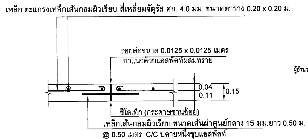
แบบขยาย ① Expansion Joint (รอยต่อเพื่อการขยายตัว) มาตราส่วน 1 : 25
