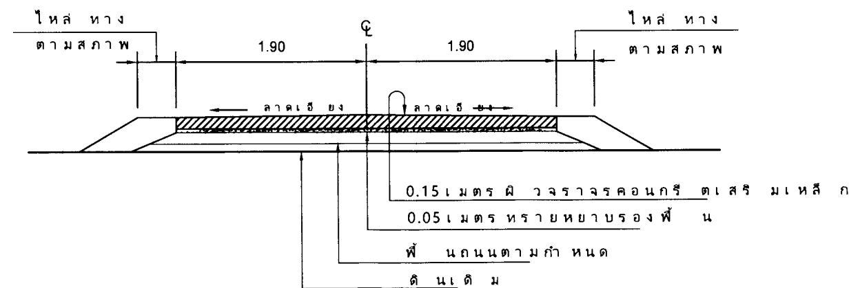
รูปตัด ก - ก มาตราส่วน 1 : 75
