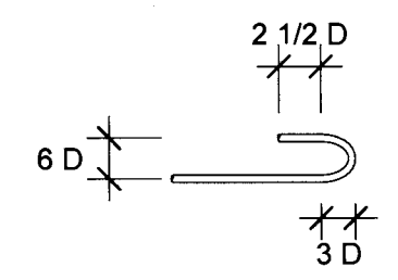
แบบแสดงการงอเหล็ก มาตราส่วน 1 : 10
