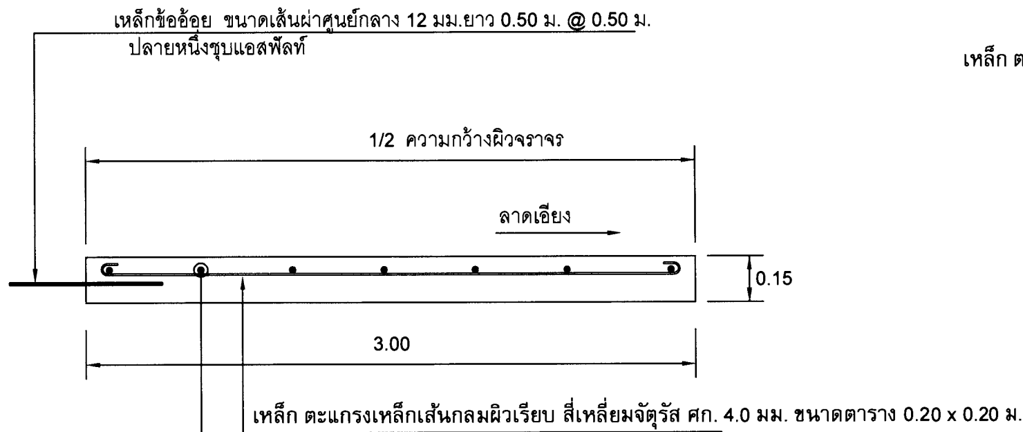
แบบขยายแสดงการผูกเหล็กตะแกรง มาตราส่วน 1 : 25
