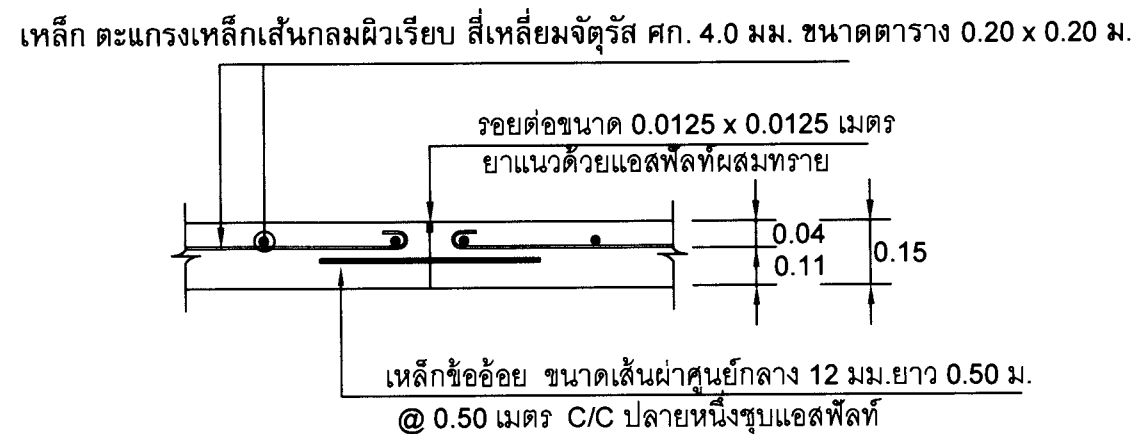
แบบขยาย ③ Longitudinal Joint (รอยต่อตามยาว) มาตราส่วน 1 : 25
