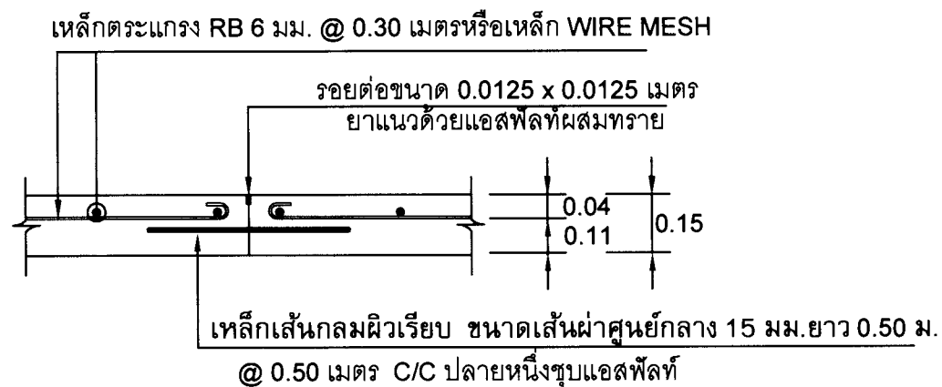
แบบขยาย ② Contraction Joint (รอยต่อเพื่อการหดตัว) มาตราส่วน 1 : 25
