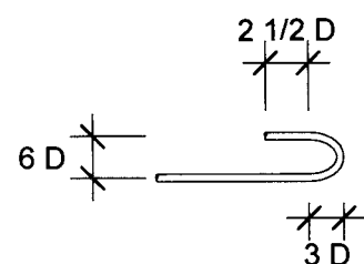
แบบแสดงการงอเหล็ก มาตราส่วน 1 : 10
