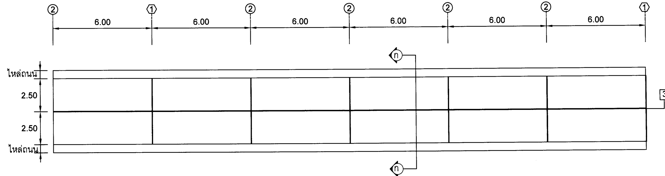
แปลนถนนคอนกรีตเสริมเหล็ก มาตราส่วน 1 : 200
