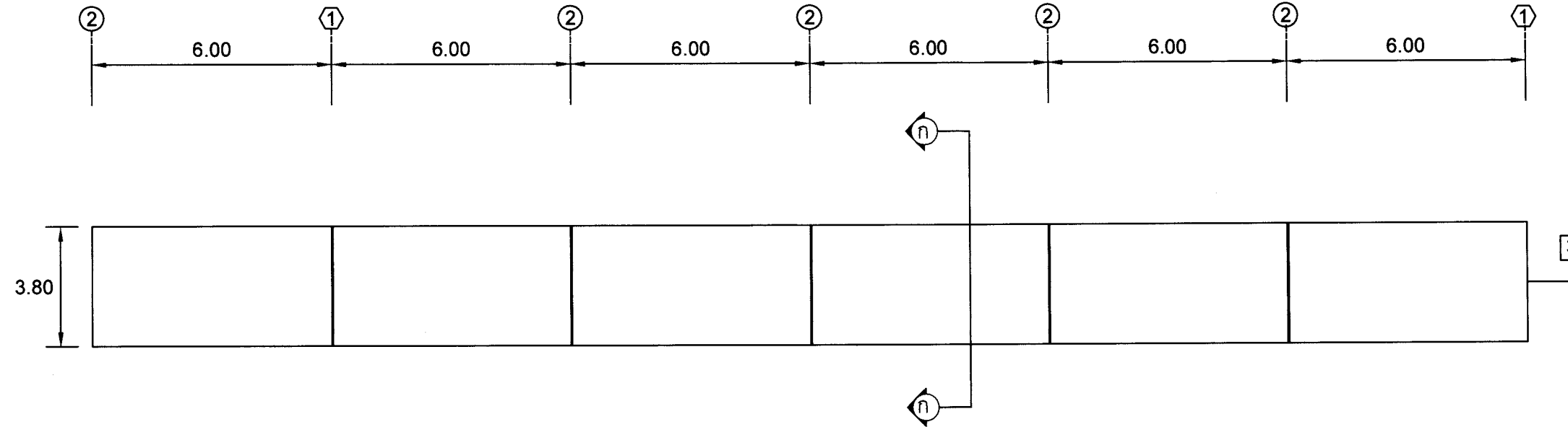
แปลนถนนคอนกรีตเสริมเหล็ก มาตราส่วน 1 : 200
